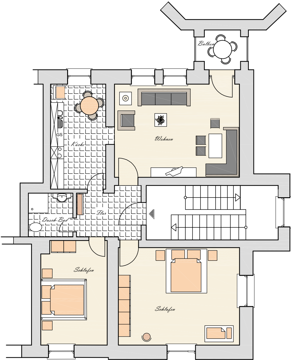
Grundriss Appartement in Binz auf Rügen "Godewind" 70.m 2
